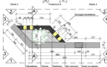
RYSUNEK TECHNICZNY DETALU - MULTI FUNKCYJONALNY MUR OPOROWY SKALA 1:75 AUTOR: KRZYSZTOF ŻYWUCKI
