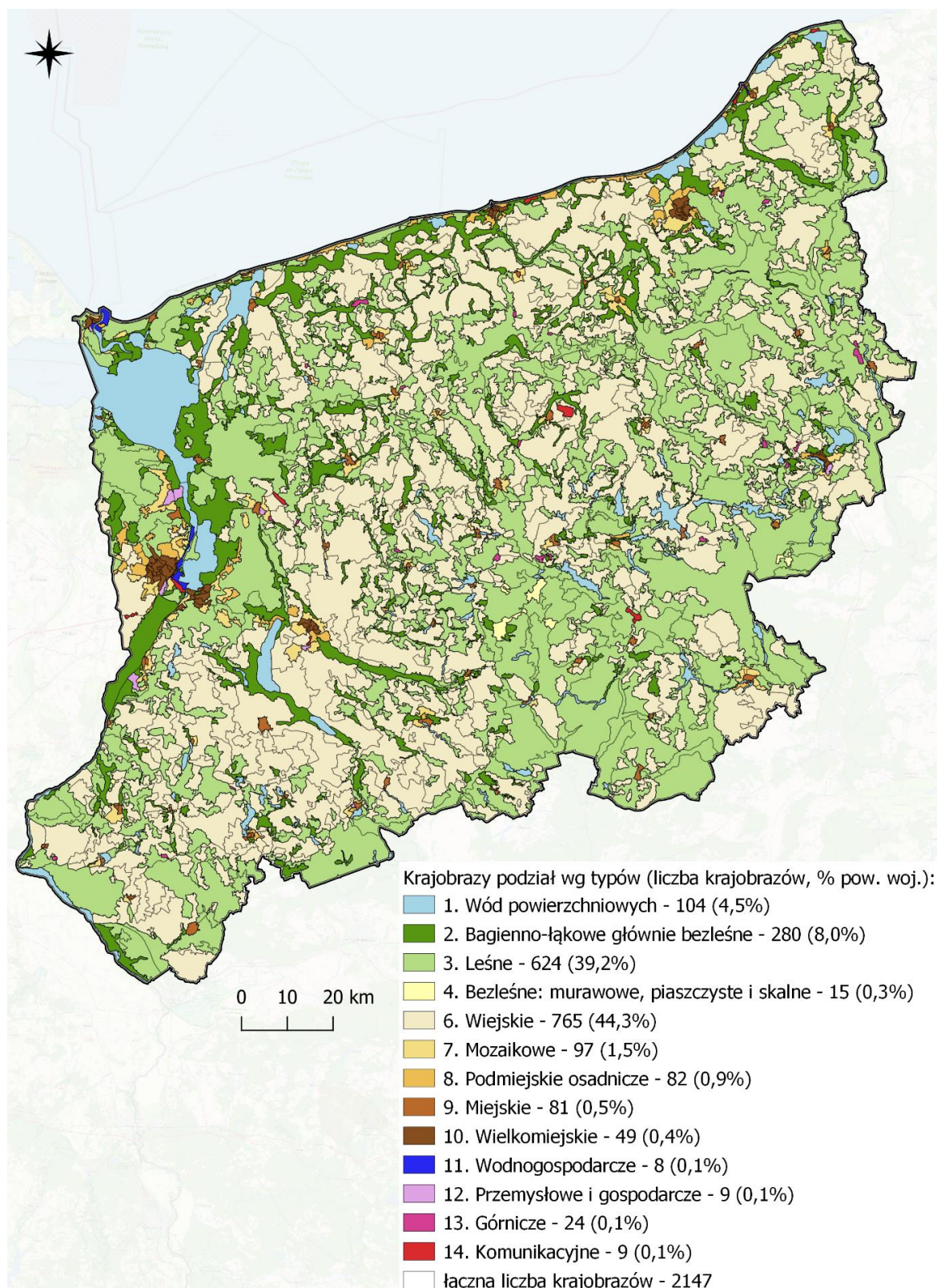
Ryc.2. Podział województwa na krajobrazy w klasyfikacji na typy pokrycia terenu
