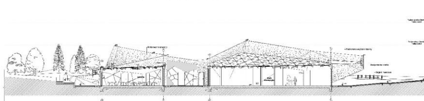
PRZEKROJ PODŁUŻNY
